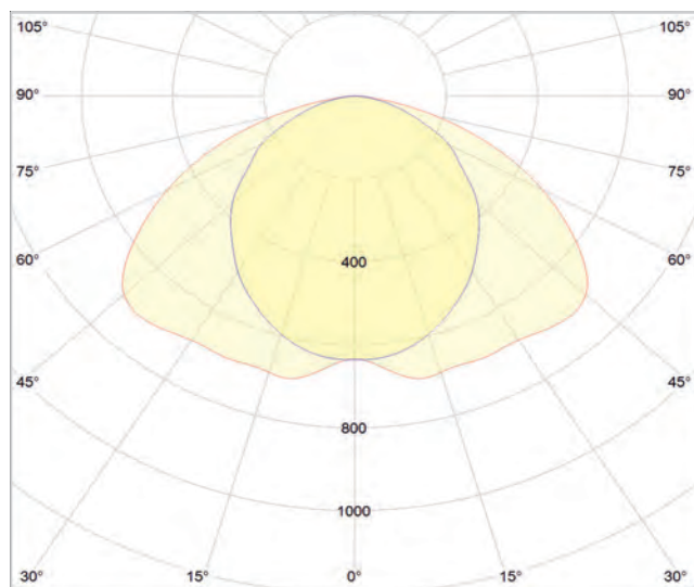
Angle de rayonnement/courbe de répartition de la lumière : 120
