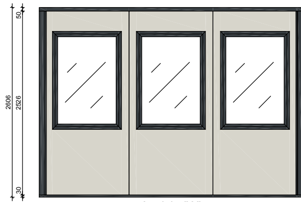
Ansicht "A"
