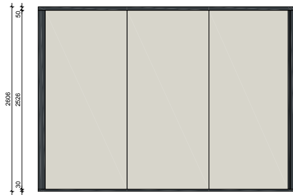
Ansicht "C"
