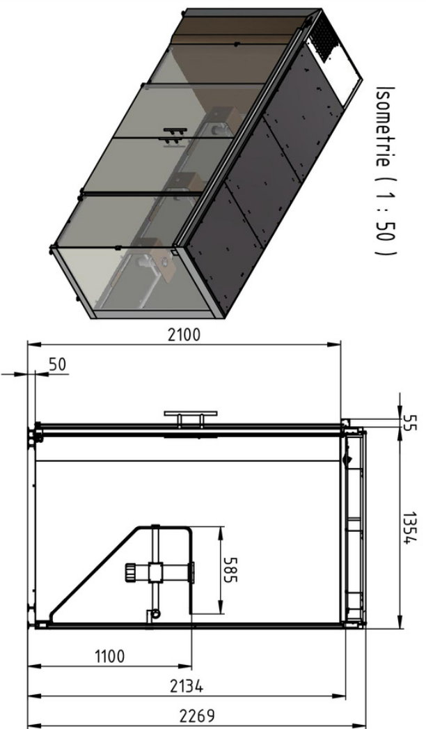
B-B ( 1 : 25 )
