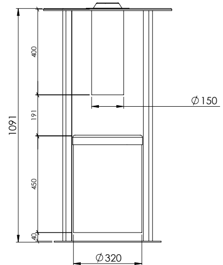
► Technische Zeichnung Rauchertisch
