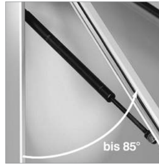
Bequemes öffnen: Flügel wird durch Gasdruckfedern bei ca 85° in Offenstellung gehalten.
