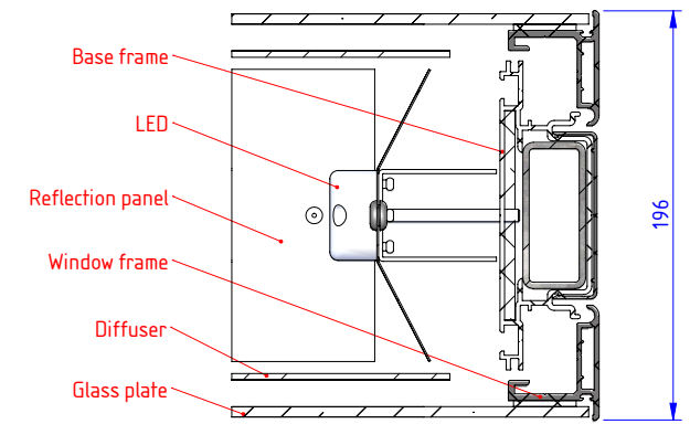
SECTION B-B (1 : 4)
