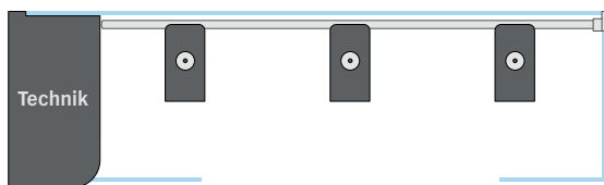
Raucherkabine ST.453-DESIGN für 12 Personen mit 3 Tischmodulen B x T x H in mm: 4530 x 1355 x 2270
