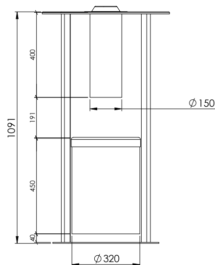
► Dessin technique de la table pour fumeurs
