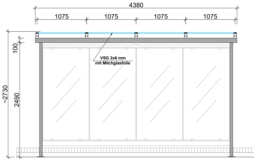
Vorderansicht
