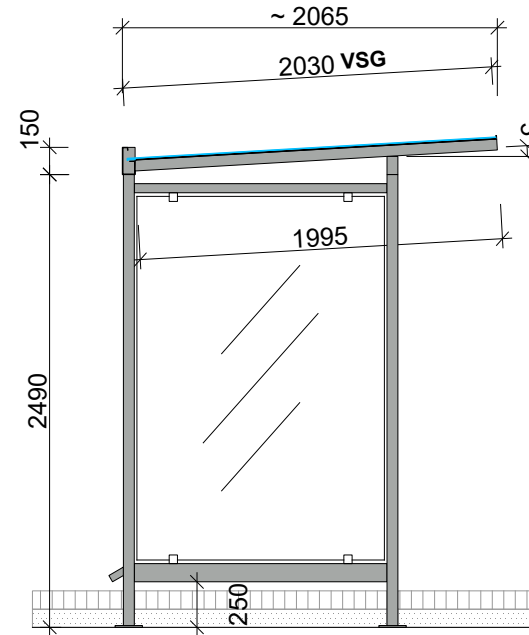
Seitenansicht
