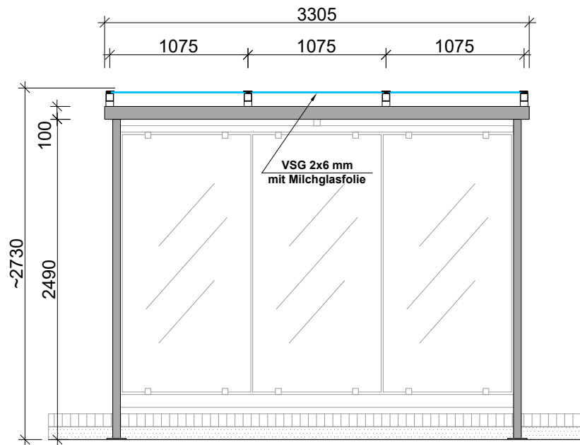
Vorderansicht
