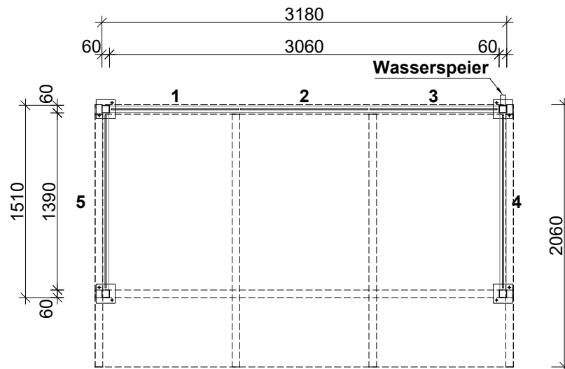
Grundriss
