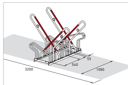
Modell 2514 XBF
