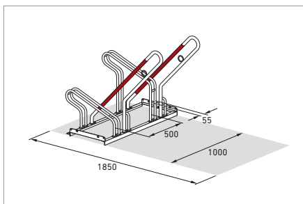
Modell 2502 XBF
